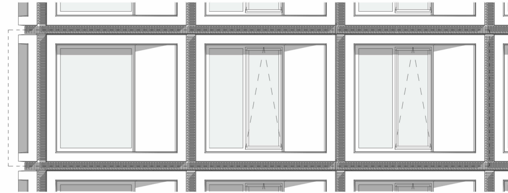
zijgevel
