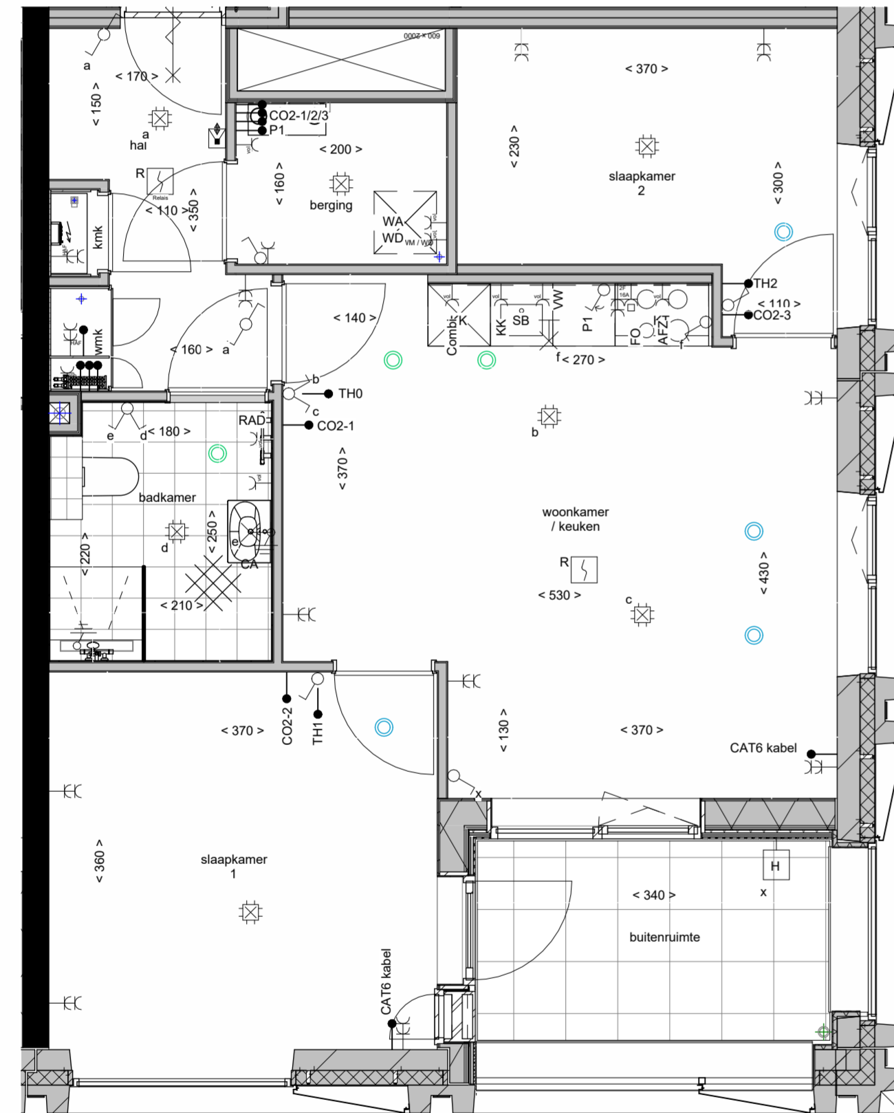
plattegrond, woningtype 01k
