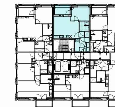
overzicht, 14e t/m 17e verdieping
