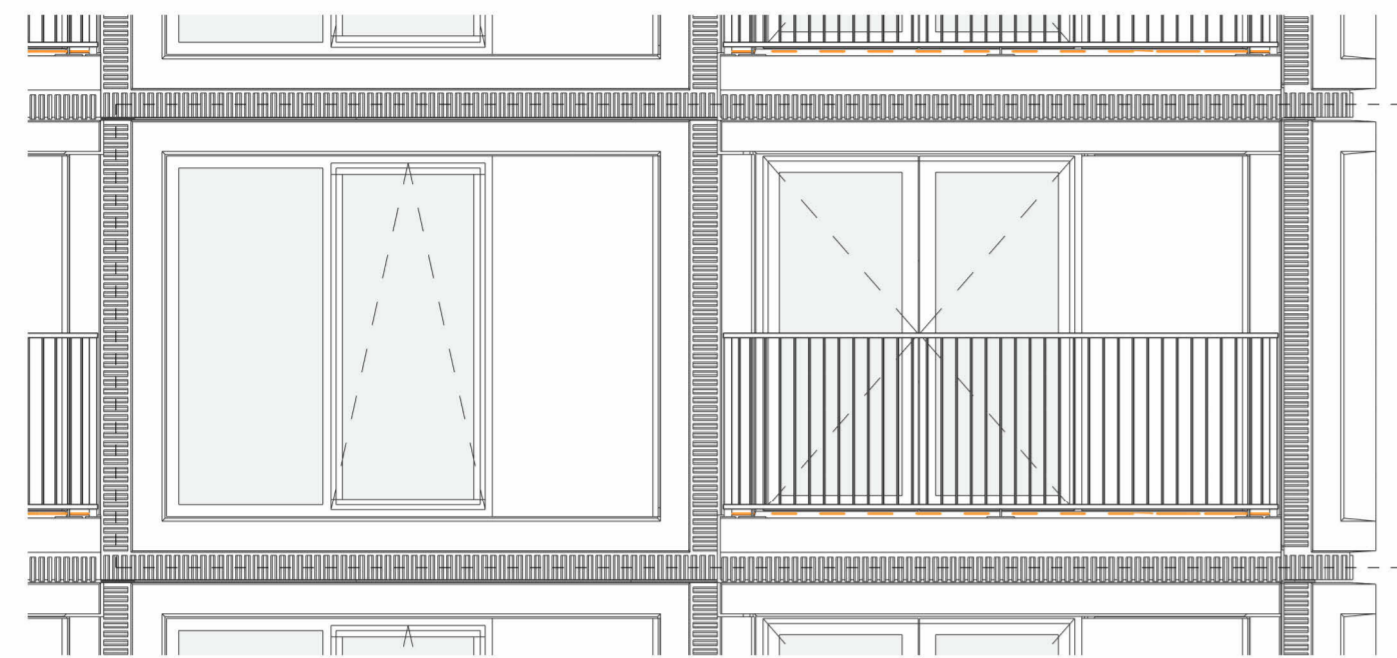
voorgevel (zuid)
