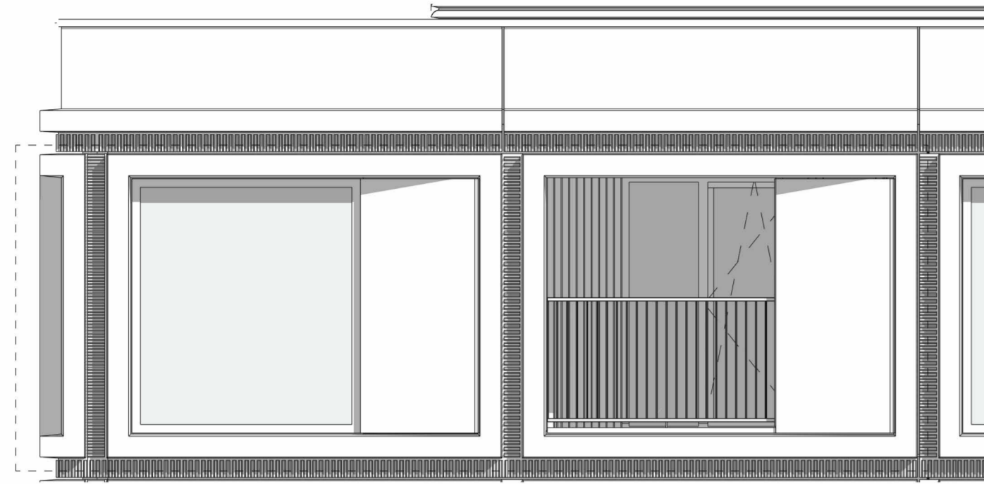
voorgevel
